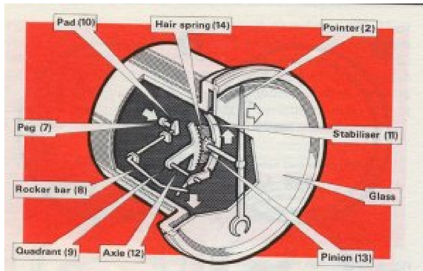
طرح نشاندهنده ساختار فشارسنج مرکب نوع دیافراگمی
