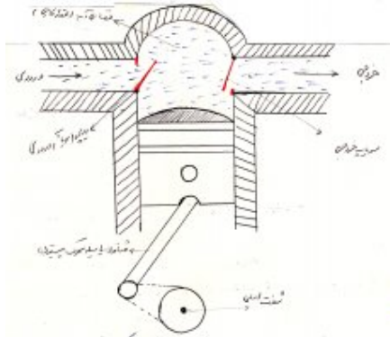
شکل (2-a) شکل ساده پمپ پیستونی نوع فشاری یکطرفه (یک عمله) در حالت عادی
