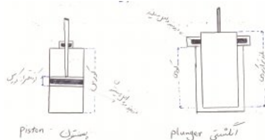
شکل 1 - تفاوت اساسی بین پیستون و انگشتی
