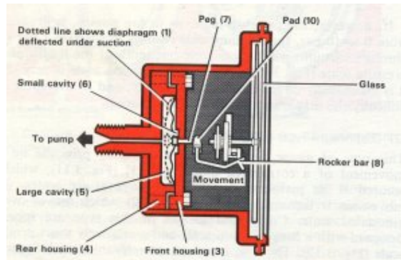
طرح نشاندهنده ساختار فشارسنج مرکب نوع دیافراگمی
