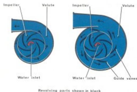
شکل (B-2) اصول و طرز کار پمپ های سنتری فیوژ
